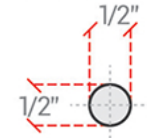
Detalles de orificio circular
